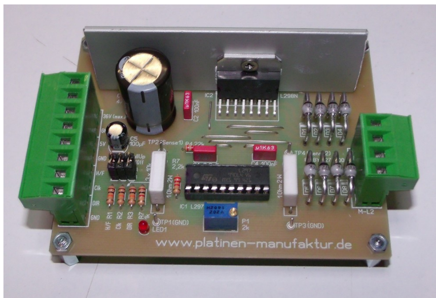
Schrittmotortreiber 9.1.2
